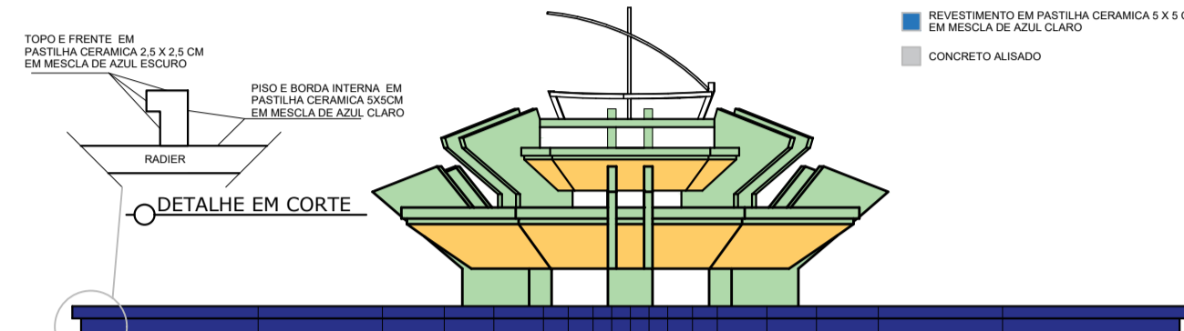
REVESTIMENTOS SEM ESCALA
