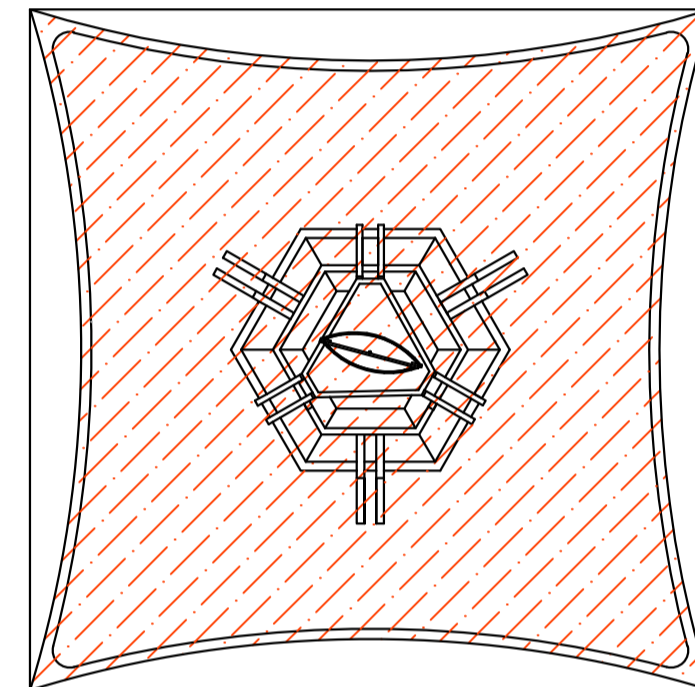
PLANTA IMPERMEABILIZAÇÃO esc. 1:200
